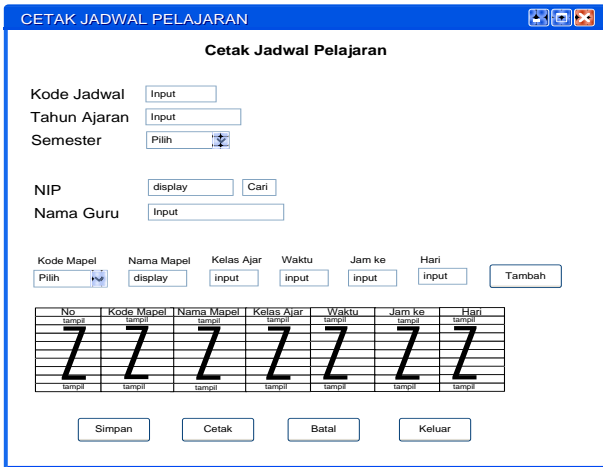
Gambar 4.24 Rancangan Layar Cetak Jadwal Pelajaran
